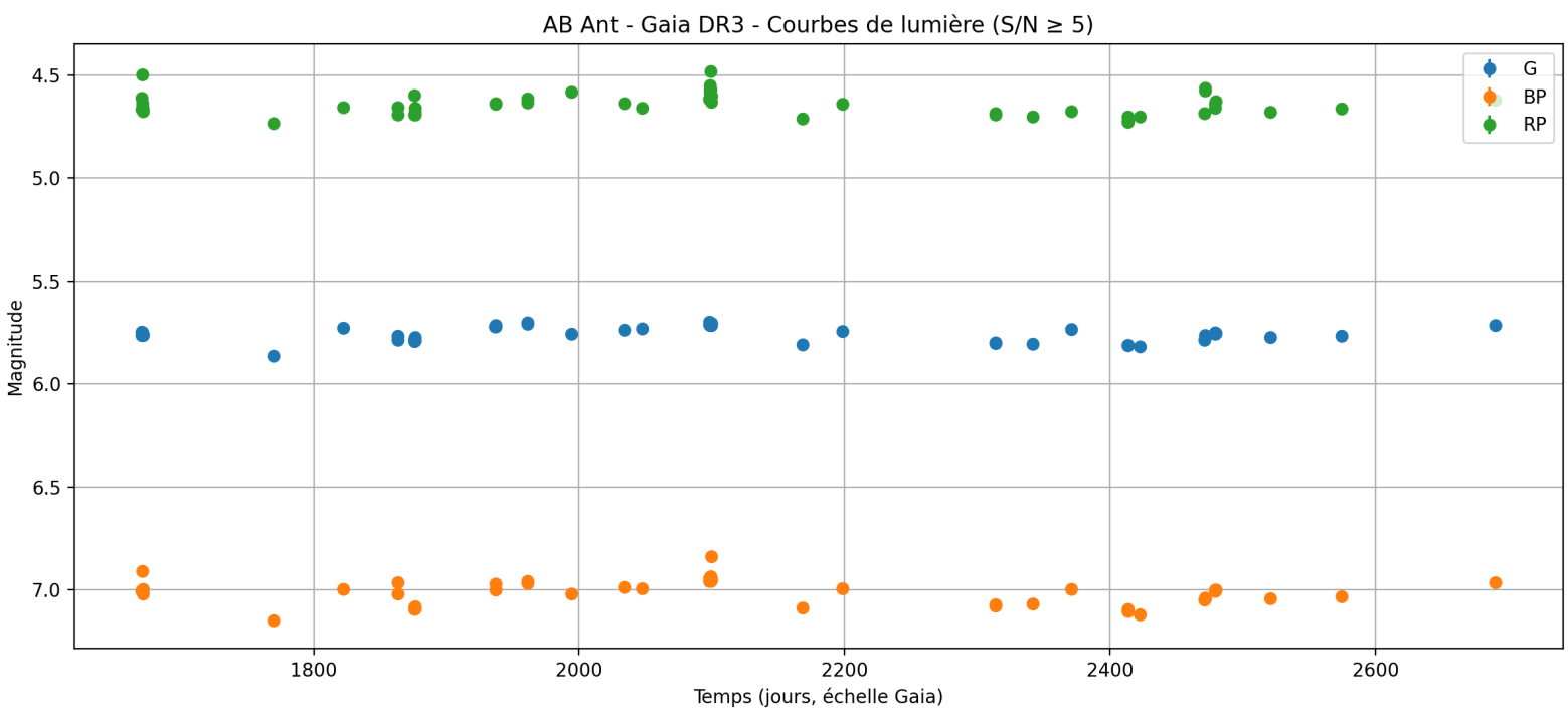
Figure 1 – Courbe de lumière Gaia pour AB Ant
