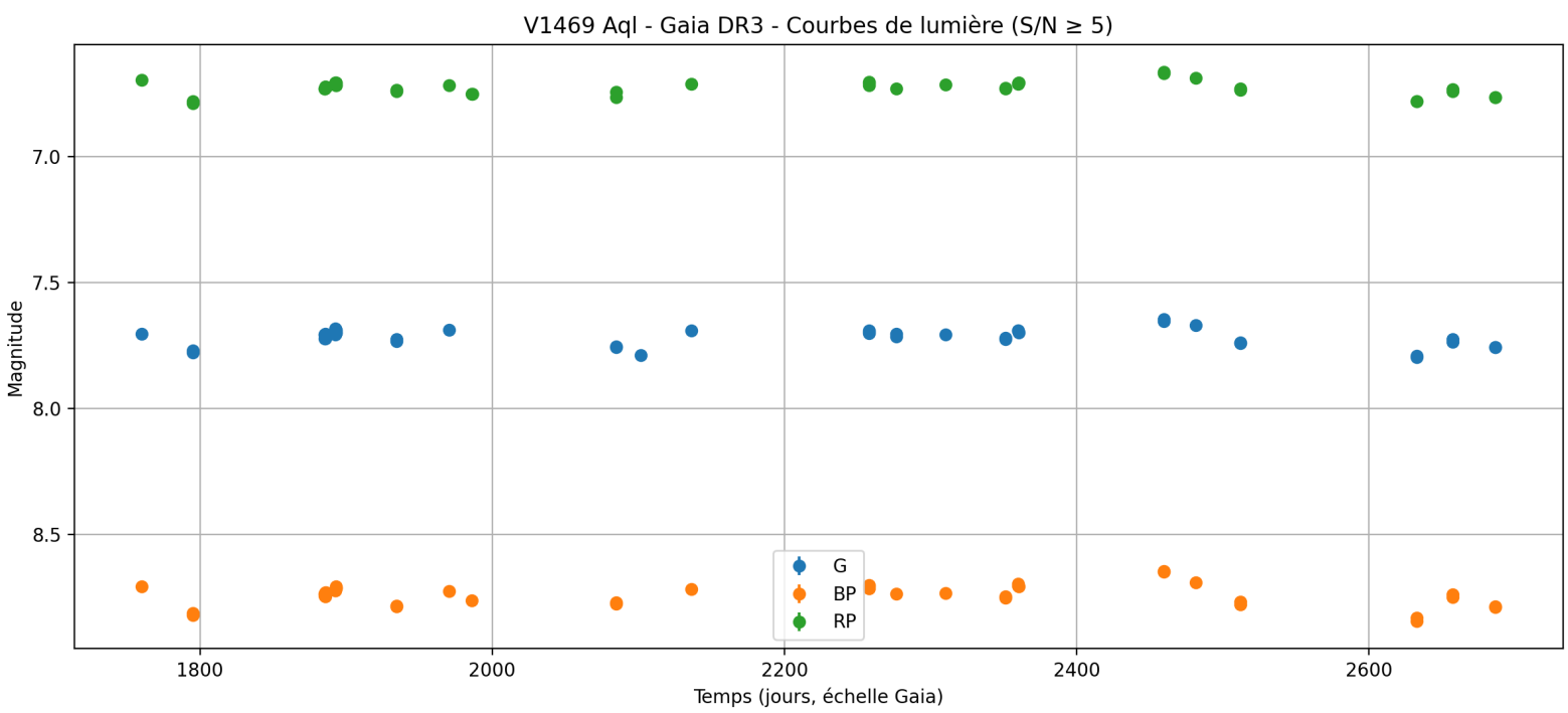
Figure 1 – Courbe de lumière Gaia pour V1469 Aql
