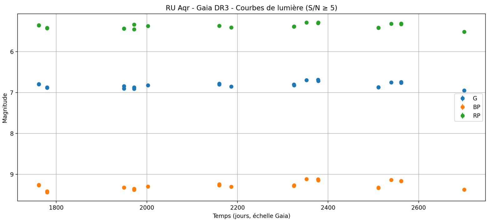
Figure 1 – Courbe de lumière Gaia pour RU Aqr
