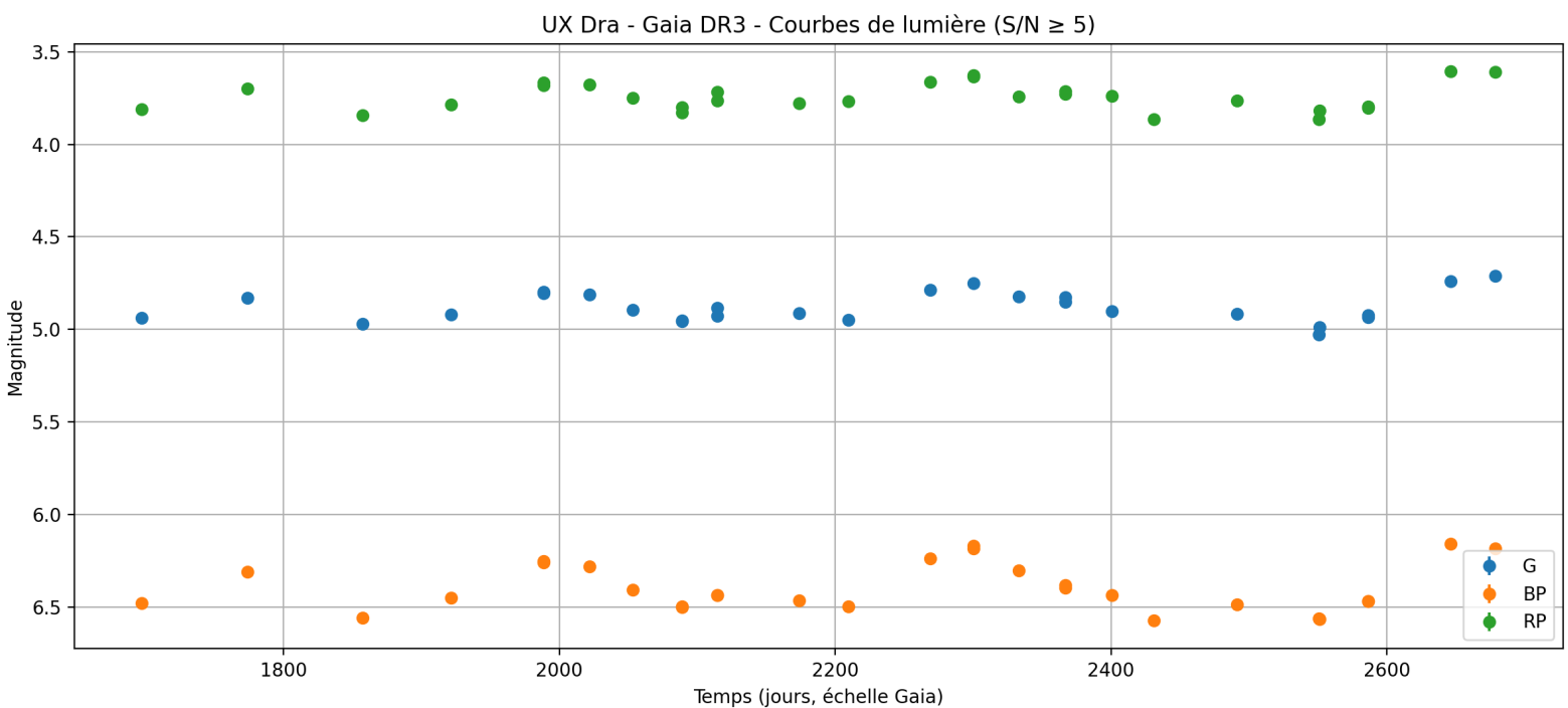
Figure 1 – Courbe de lumière Gaia pour UX Dra
