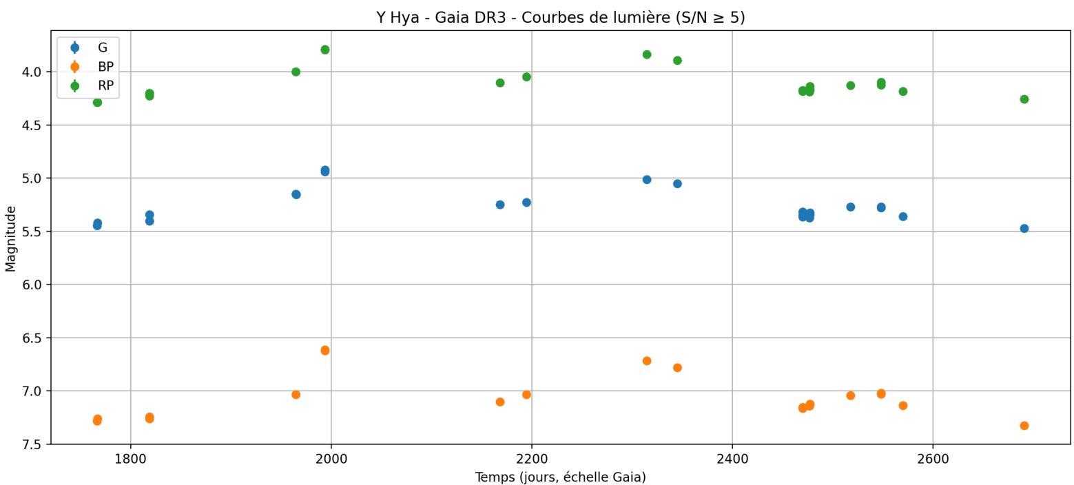
Figure 1 – Courbe de lumière Gaia pour Y Hya
