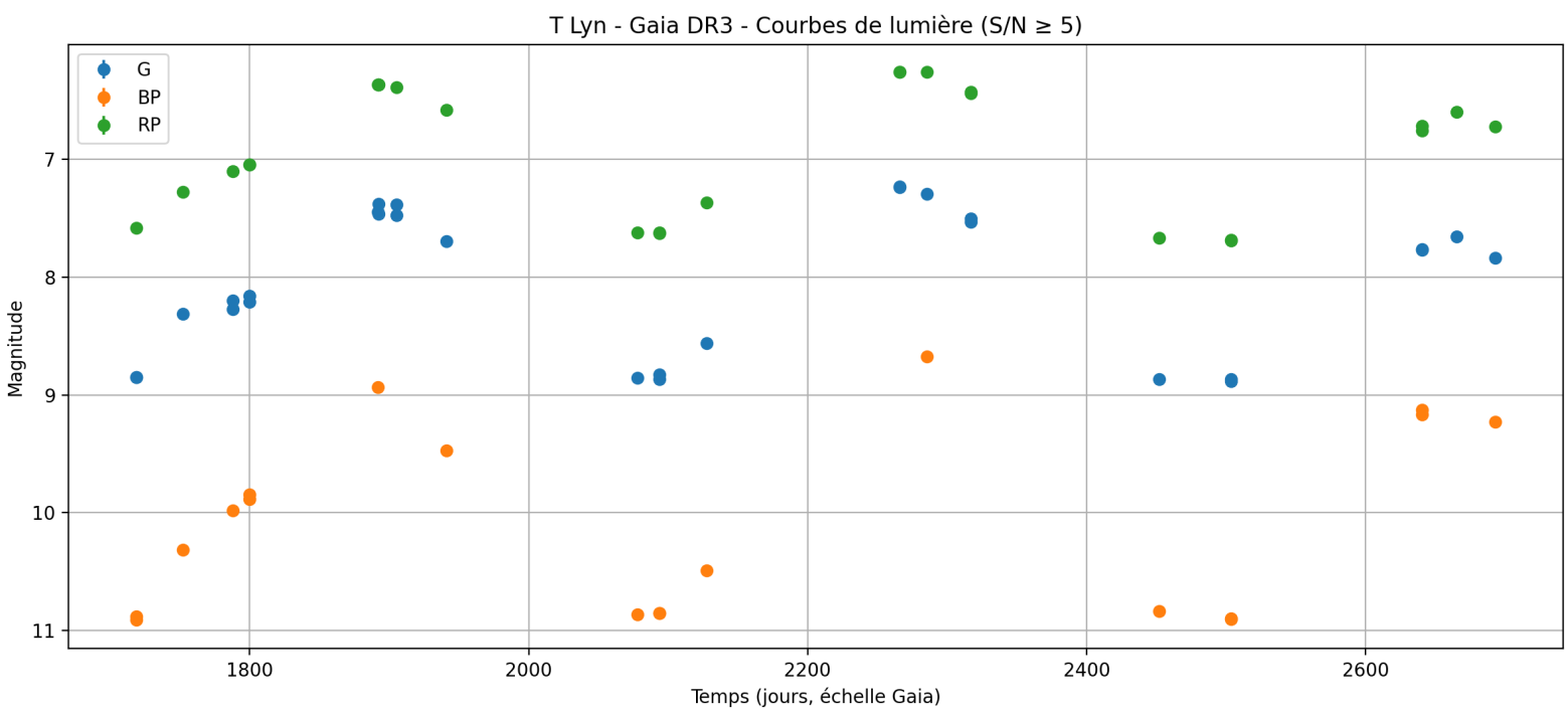
Figure 1 – Courbe de lumière Gaia pour T Lyn
