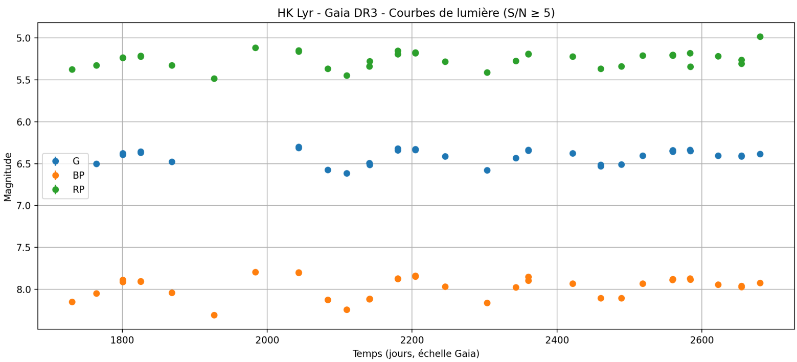
Figure 1 – Courbe de lumière Gaia pour HK Lyr
