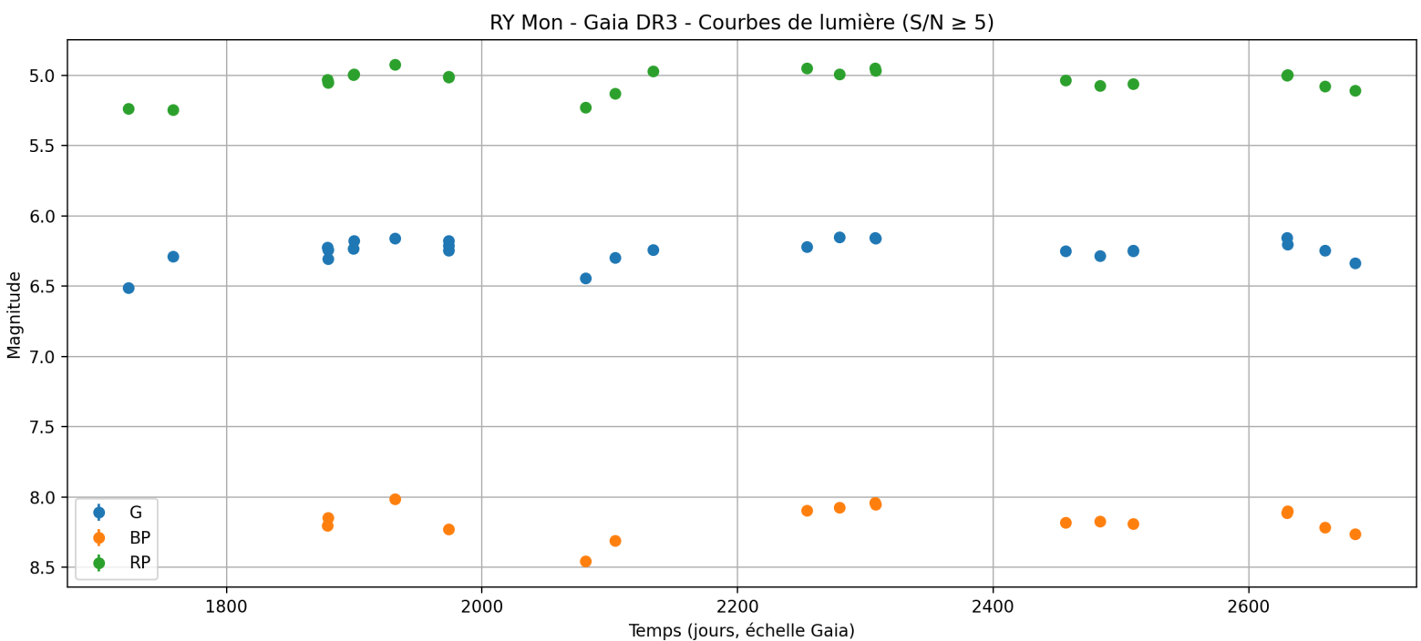
Figure 1 – Courbe de lumière Gaia pour RY Mon
