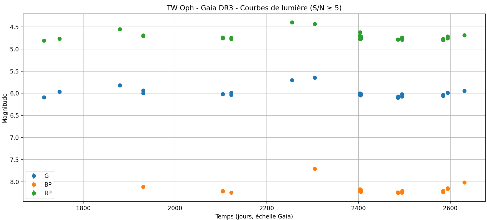
Figure 1 – Courbe de lumière Gaia pour TW Oph
