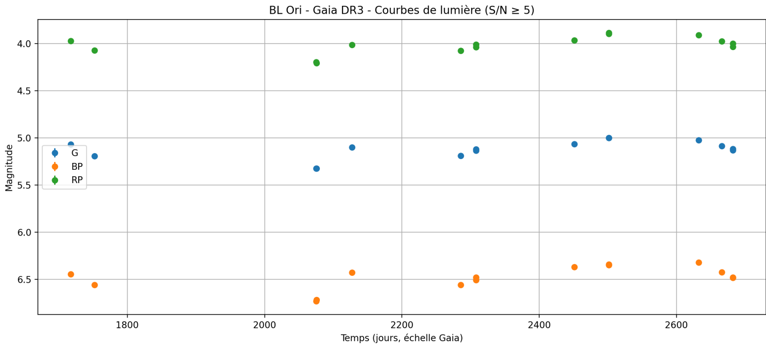
Figure 1 – Courbe de lumière Gaia pour BL Ori
