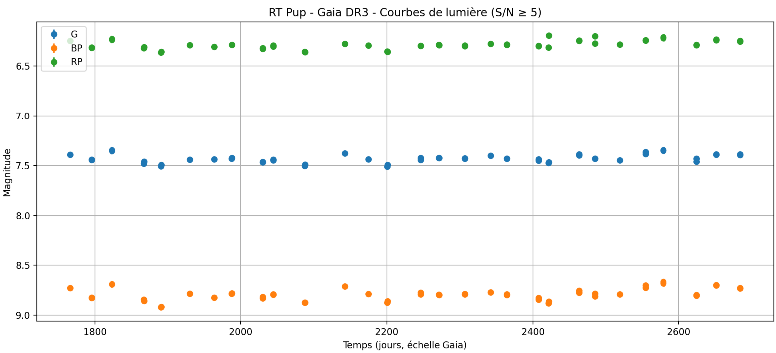
Figure 1 – Courbe de lumière Gaia pour RT Pup
