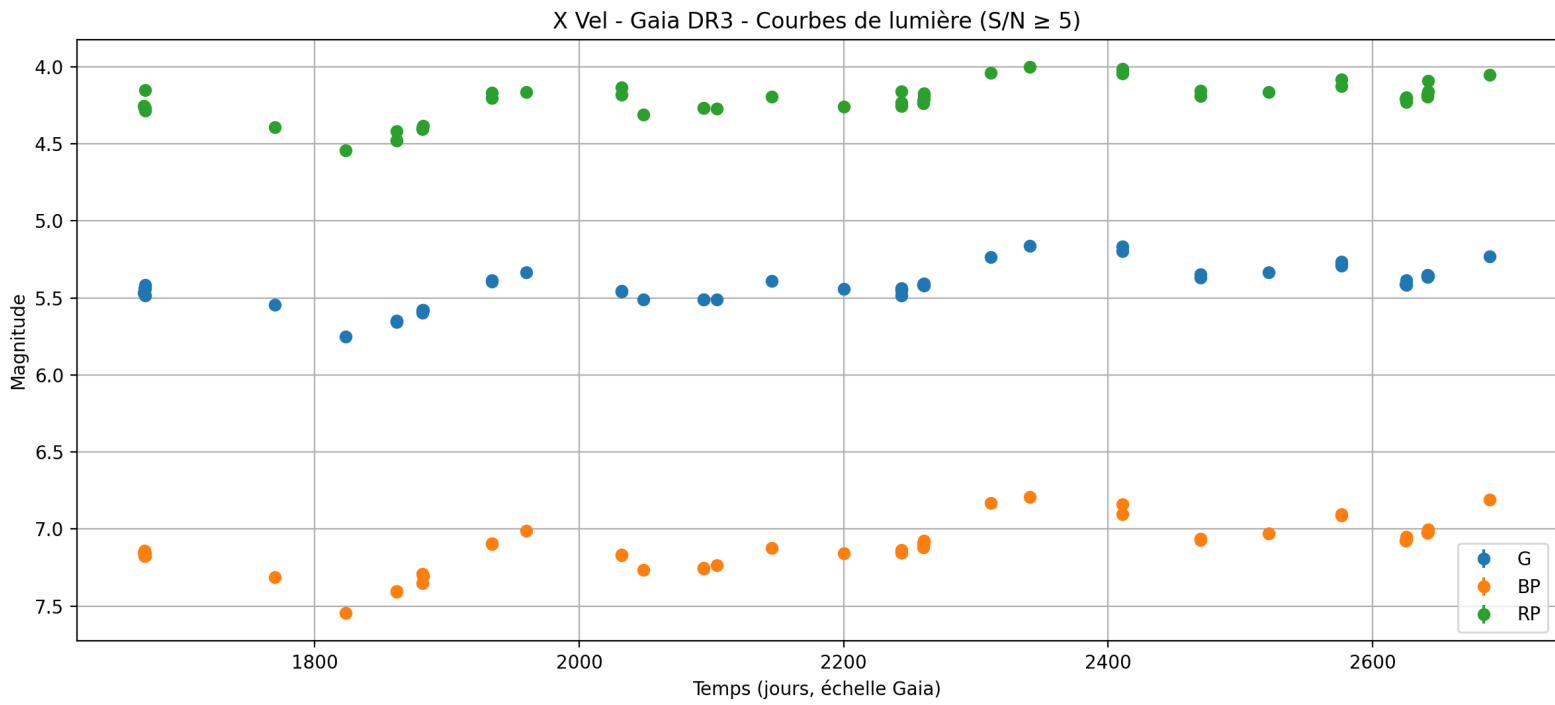
Figure 1 – Courbe de lumière Gaia pour X Vel
